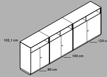
Kombischränk Regal/Flügeltüren, 2,5 Ordnerhöhen Combined cabinet, shelf/hinged doors, 2,5 files high
