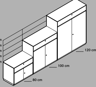
Kombischränk Schubfach/Flügeltüren, 1,5 bis 3,5 Ordnerhöhen Combined cabinet, large drawer/hinged doors, 1,5 to 3,5 files high
