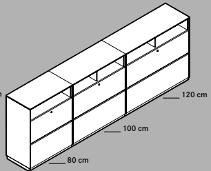
Kombischränk Regal/Hängehefter, 2,5 Ordnerhöhen Combined cabinet, shelf/filing, 2,5 files high
