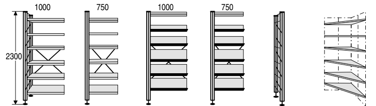
2300 mm hoch, komplett mit Böden
