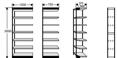
2600 mm hoch und 7 Fachböden
